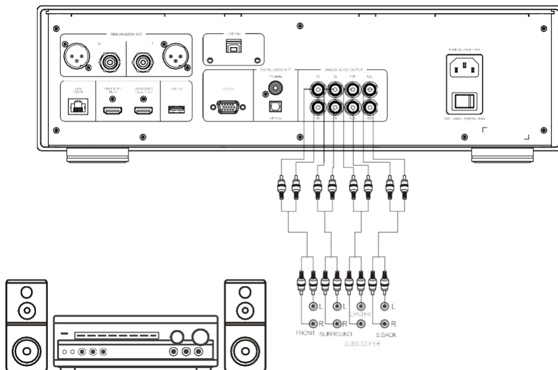
Přijímač/zesilovač s 7.1kanálovým audio vstupem
